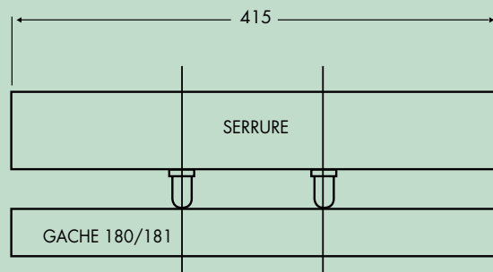
Serrure 70182
