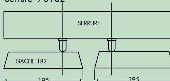
Serrure 70182
