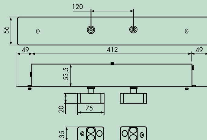
Serrure 70183 i
